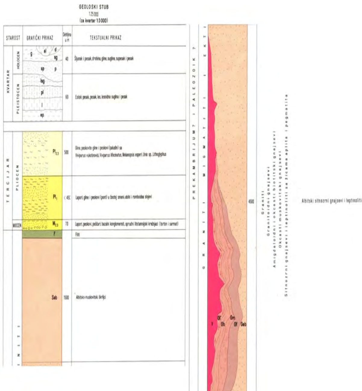
Слика 6: Геолошки стуб КО Марковац
