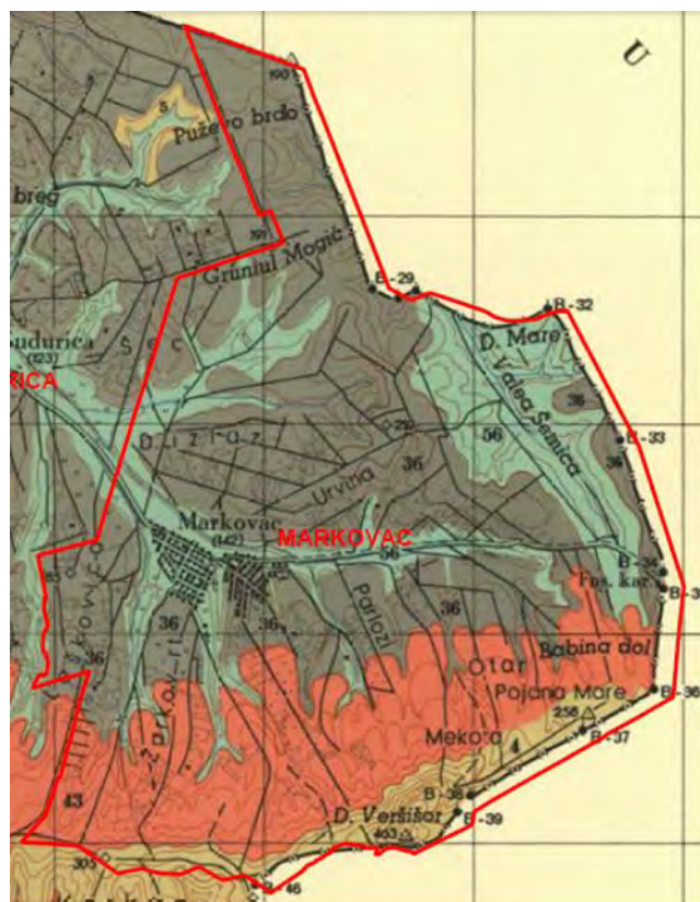
Слика 7: Педолошка карта КО Марковац
